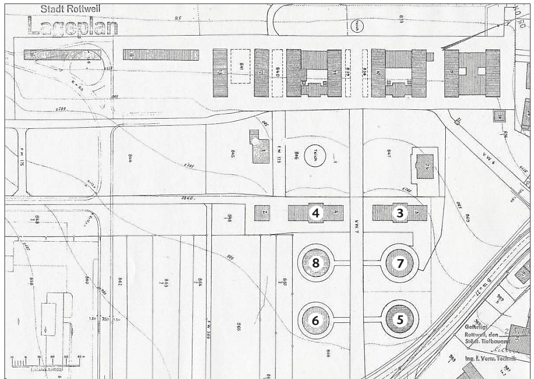
Lageplan der Königlichen Saline Wilhelmshall mit nummerierten Gebäuden Vorlage: Stadtverwaltung Rottweil, Tiefbauamt
